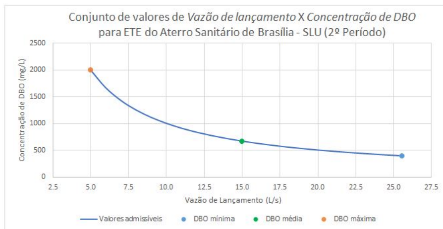
Figura 01 - Gráfico de conjunto de valores admissíveis para a vazão de lançamento e concentração de DBO efluente
