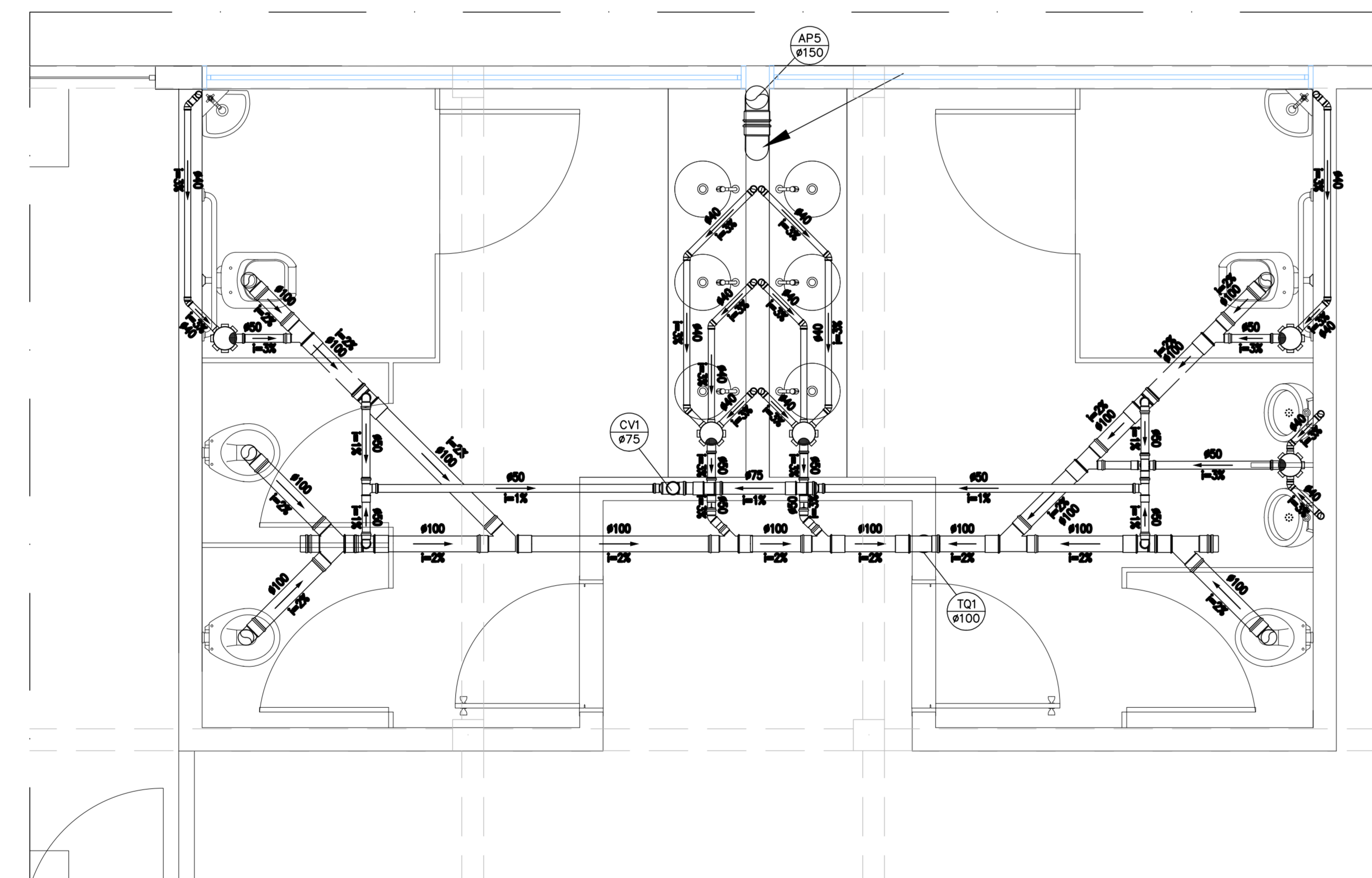
DETALHE 9 Esc. 1:25
