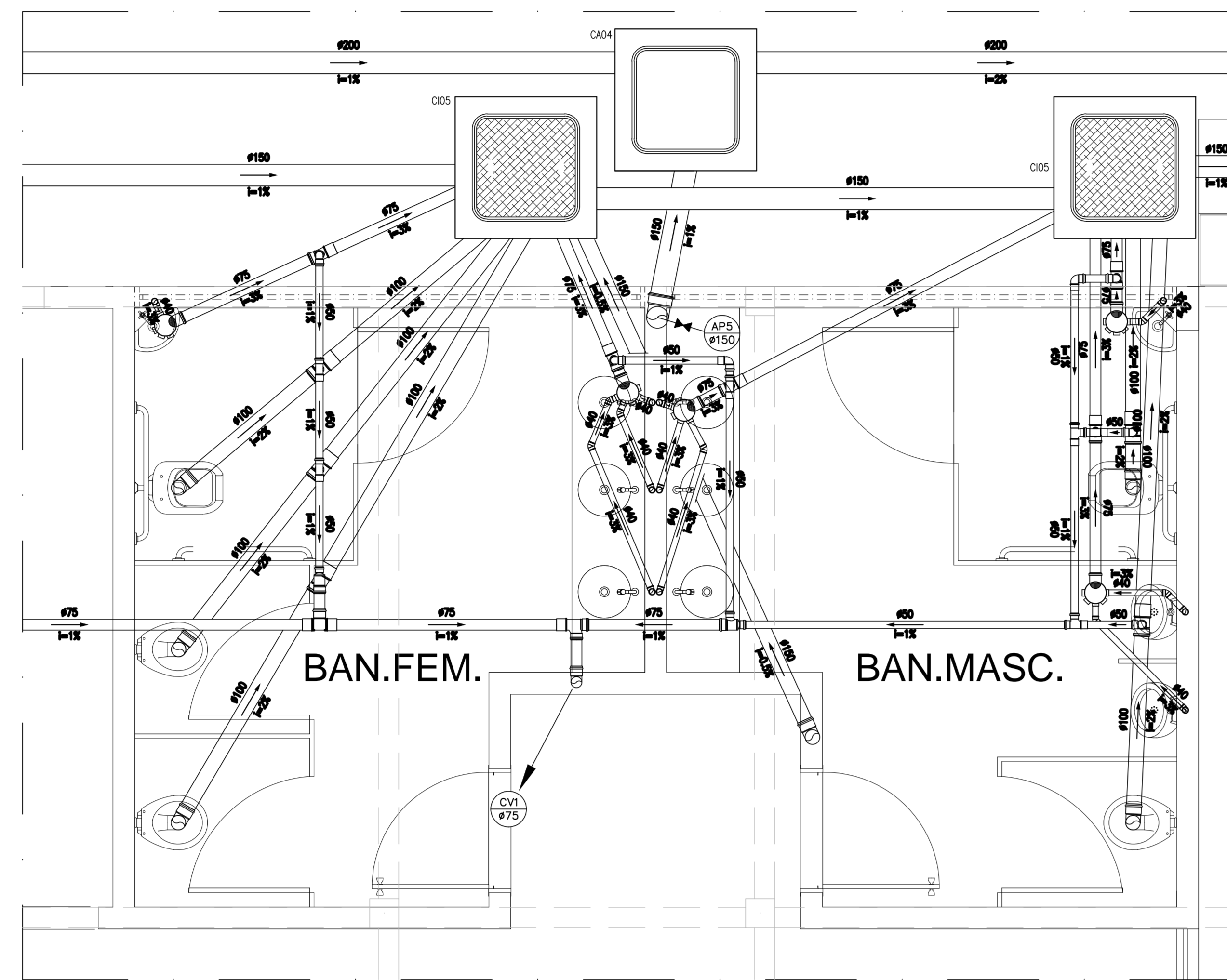
DETALHE 8 Esc. 1:25
