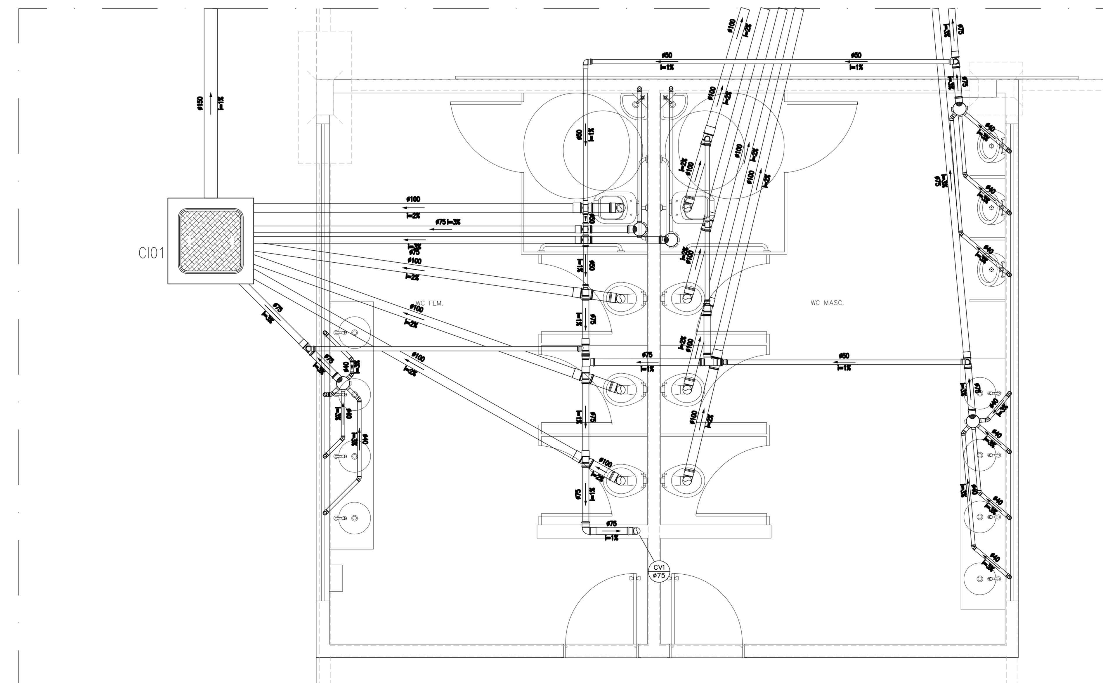
DETALHE 10 Esc. 1:25
