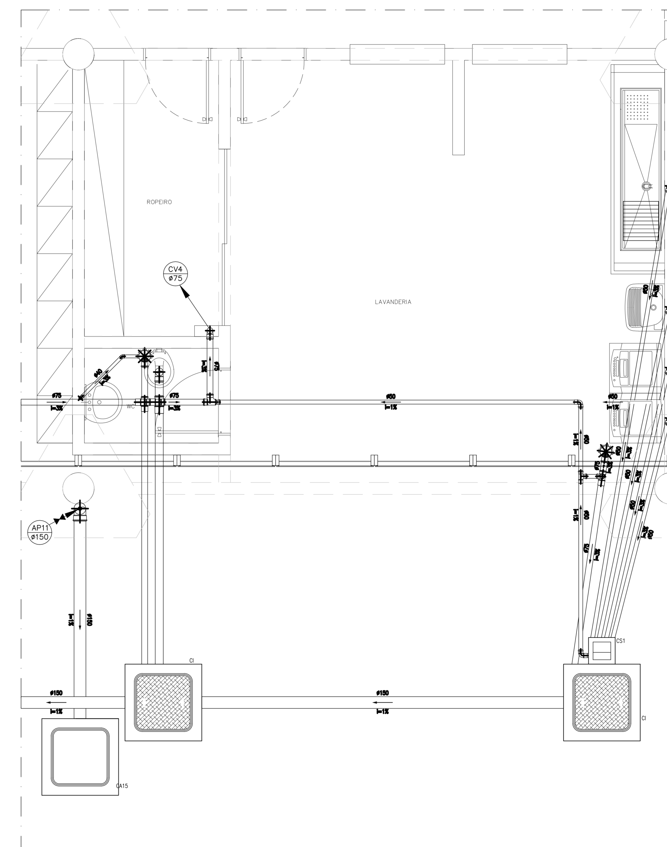
DETALHE 6 ESC. 1/25
